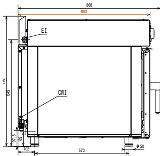
Zij aanzicht
