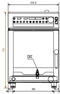
Front aanzicht
